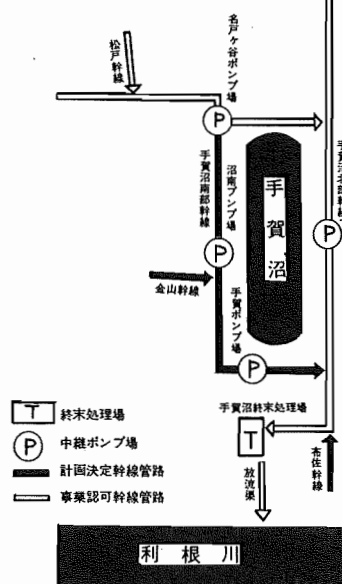
手賀沼流域下水道系統図
