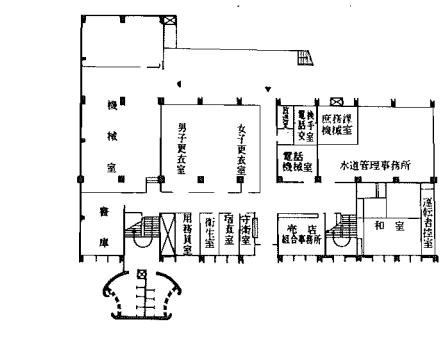
地階平面図
