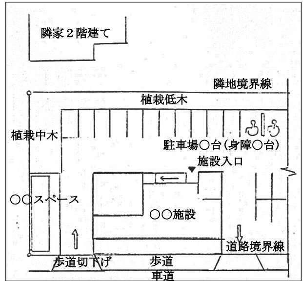
例：配置図
