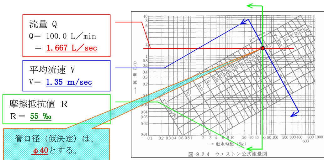
流量線図の見方の例
