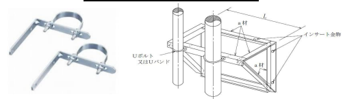
給水配管の支持金物
