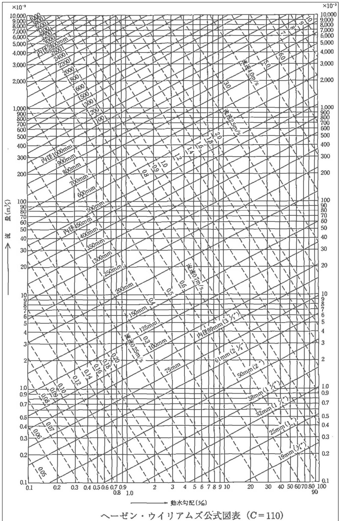
ハーゼン・ウィリアムズ公式流量図
