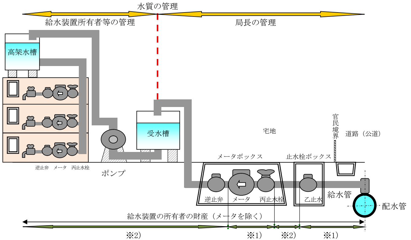
貯水槽給水の水質管理、修繕区分の概要図
