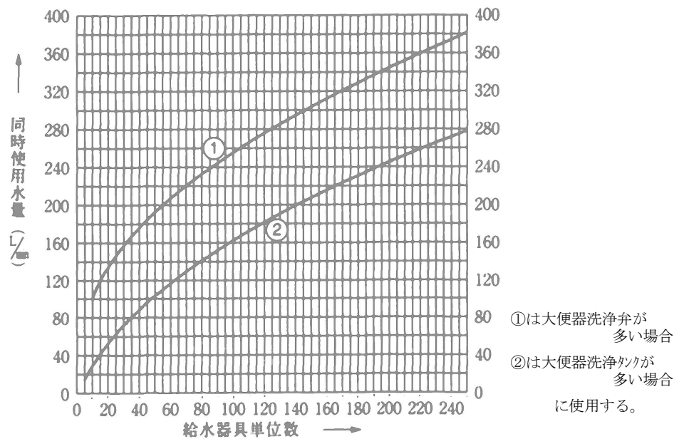
器具給水負荷単位による計画瞬時最大流量 線図
