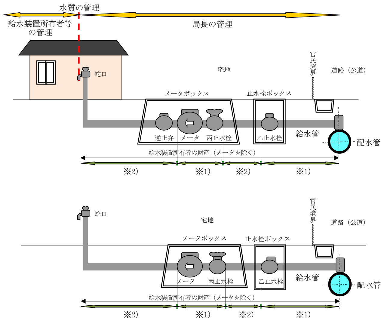
一般給水の水質管理、修繕区分の概要図
