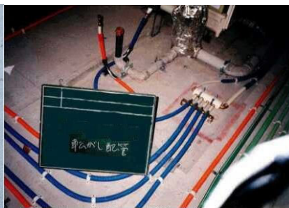
ヘッダー廻りの給水配管 [床下騒音発生現場 (竣工後3年)]
