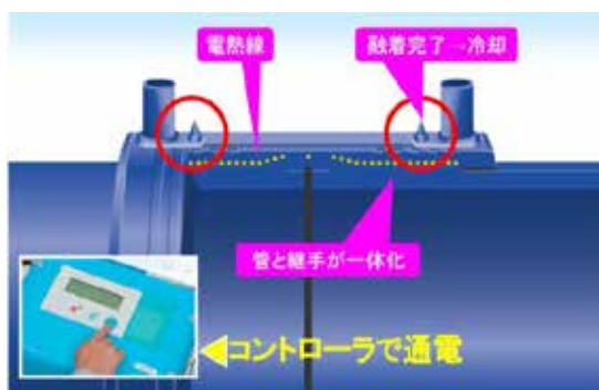
融着継手の構造(配水用ポリエチレン管)
