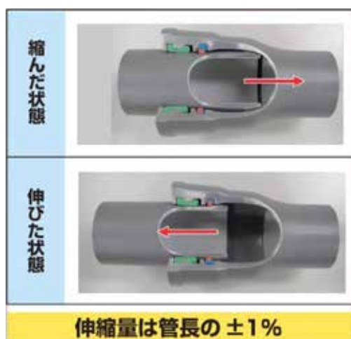
耐震継手の構造(ダクタイル鋳鉄管)
