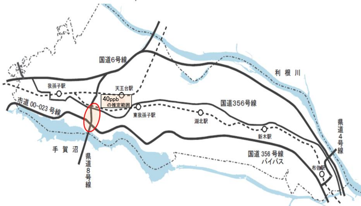
図1-10 窒素酸化物濃度等濃度線図(令和元年(2019年)12月調査)単位:ppb*
