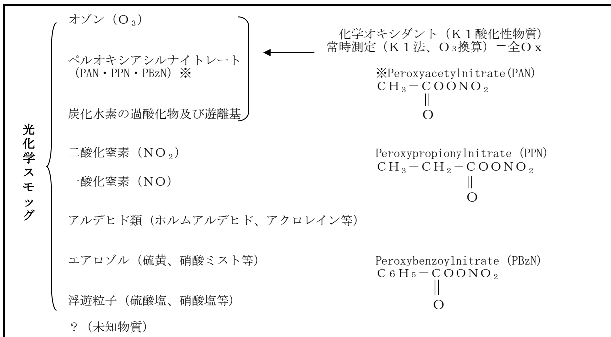
図1-4 光化学スモッグの有害成分
