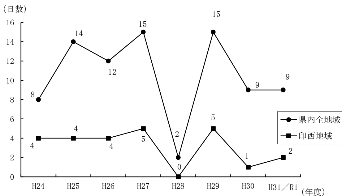
図1-7 光化学スモッグ注意報発令日数の経年変化
