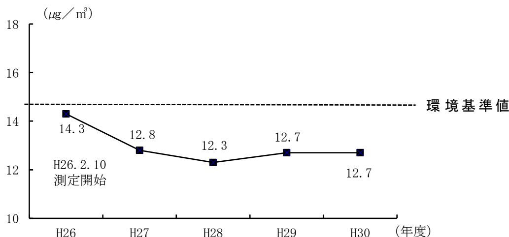
図1-3 微小粒子状物質の年平均値の経年変化 (我孫子湖北台測定局)
