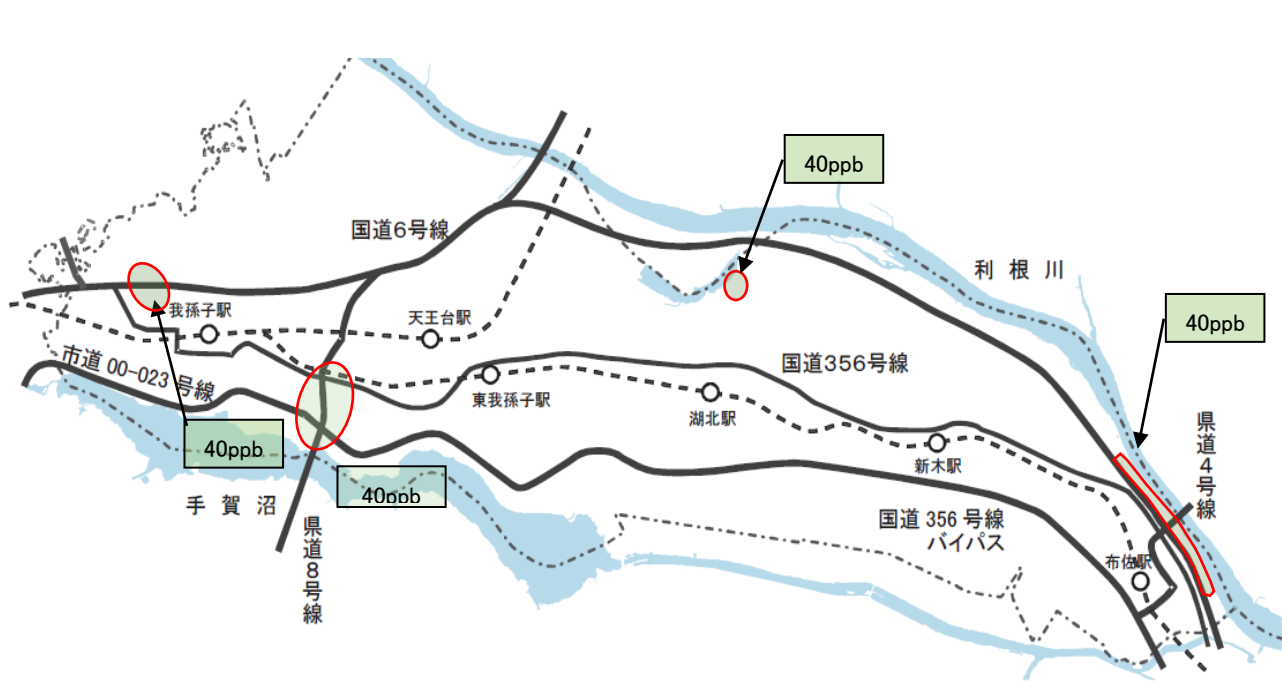
図1-10 窒素酸化物濃度等濃度線図(平成30年(2018年)12月調査)単位: ppb*
