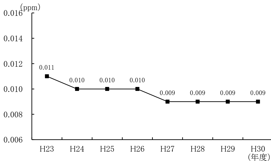
図1-1 二酸化窒素 (NO 2 ) の年平均値の経年変化 (我孫子湖北台測定局)
