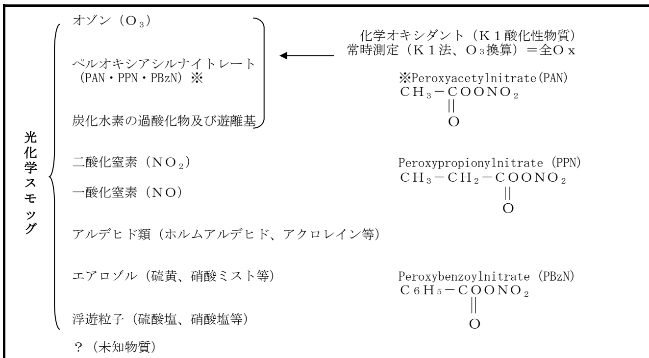
図1-4 光化学スモッグの有害成分
