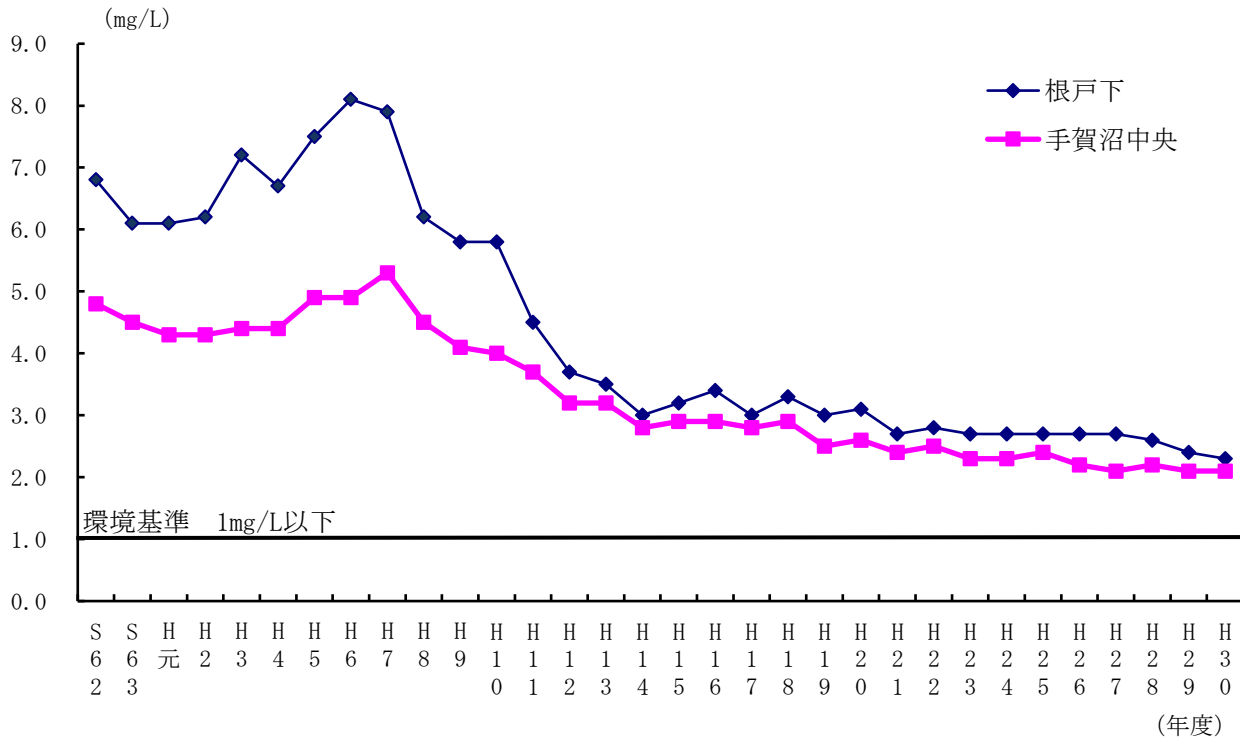
図1-6 手賀沼の全窒素の経年変化 (年平均値)
