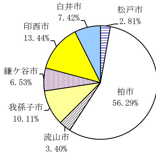
図1-3-1 市別の流域面積 (割合)
