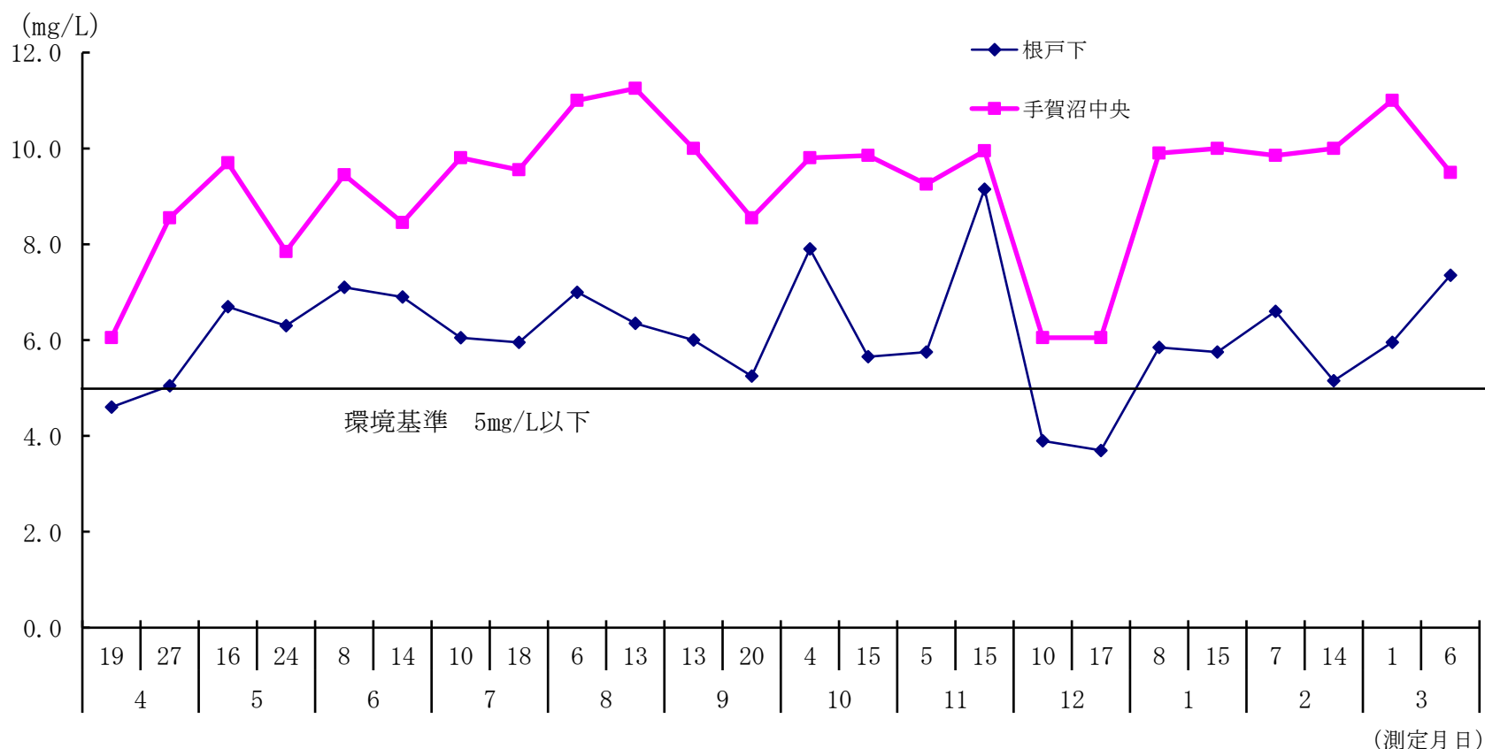
図1-8 手賀沼のCODの月別変化（平成30年度）
