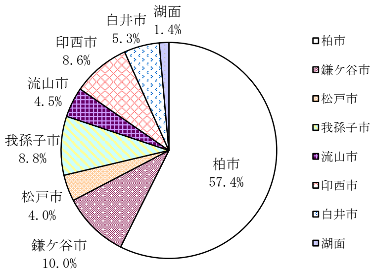
図 1-1 1 市等別汚濁負荷量
