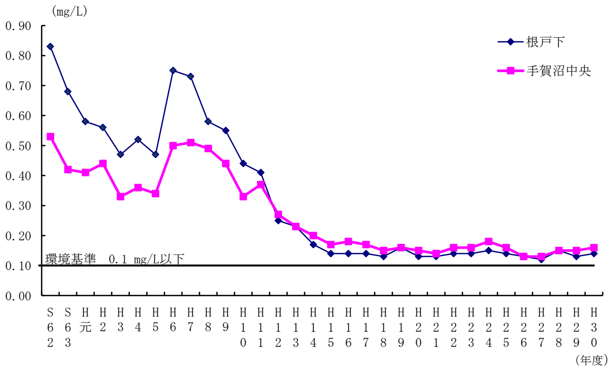
図1-7 手賀沼の全リンの経年変化 (年平均値)
