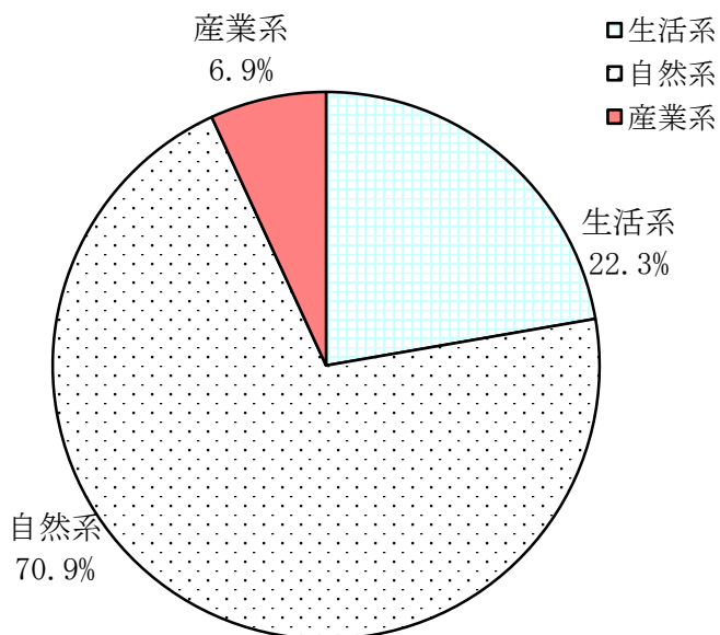
図 1-1 2 発生源別汚濁負荷量
