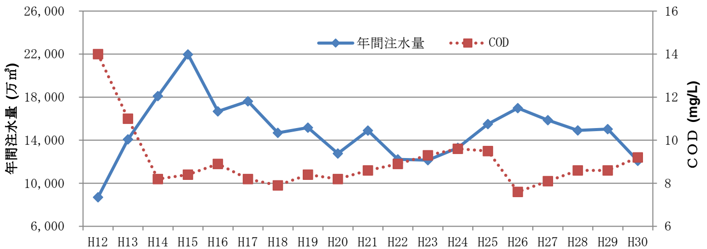
図1-13 北千葉導水年間注水量及びCOD
