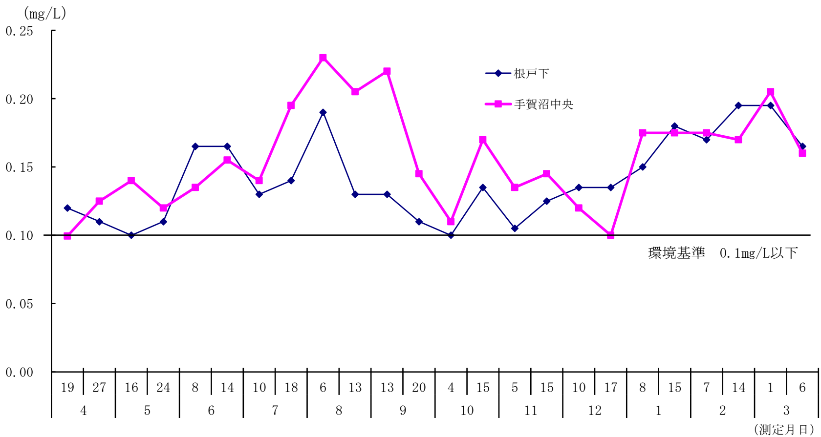
図1-10 手賀沼の全リンの月別変化 (平成30年度)
