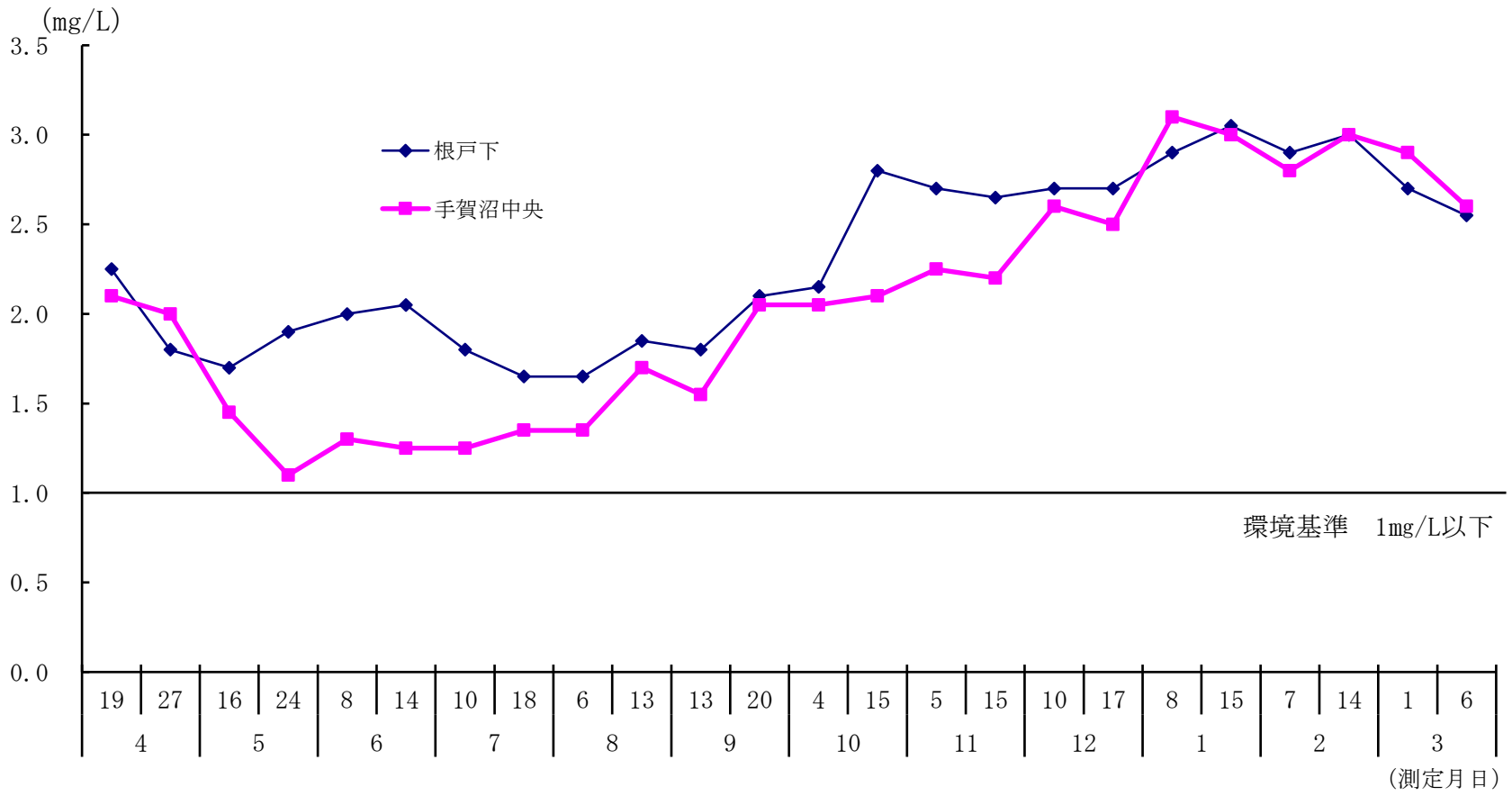
図1-9 手賀沼の全窒素の月別変化 (平成30年度)
