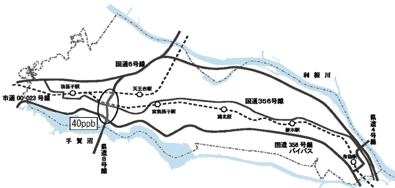
図1-8 窒素酸化物濃度等濃度線図(平成27年1月調査) 単位: ppb
